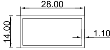
مستطيل (1.1*14*28) ملم الرقم التسلسلي للصنف: H28X14X1.1 الوزن: 0.238:(Kg/m)
