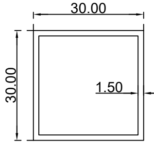
مربع (1.5*30*30) ملم الرقم التسلسلي للصنف: FG30X30X1.5 الوزن: 0.465:(Kg/m)
