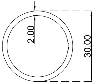
انبوب دائري مجوف (2*30) ملم الرقم التسلسلي للصنف: BLT3577 الوزن 0.477:(Kg/m)
