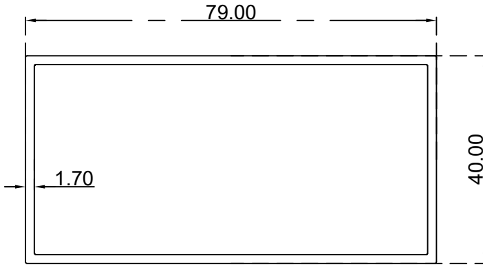
مستطيل (1.7*40*79) ملم الرقم التسلسلي للصنف: FG79X40X1.70 الوزن (Kg/m): 1.069
