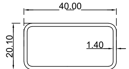
مستطيل (1.4*20*40) ملم الرقم التسلسلي للصنف: FG40X20.1X1.4 الوزن: 0.408:(Kg/m)
