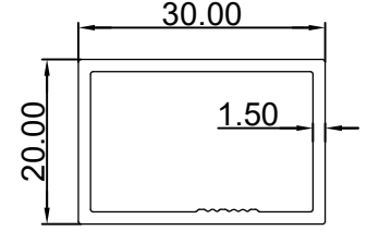
مستطيل (1.5*20*30) ملم الرقم التسلسلي للصنف: BLT3690 الوزن: 0.387:(Kg/m)
