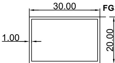
مستطيل (1*20*30) ملم الرقم التسلسلي للصنف: FG30X20X1 الوزن: 0.261:(Kg/m)
