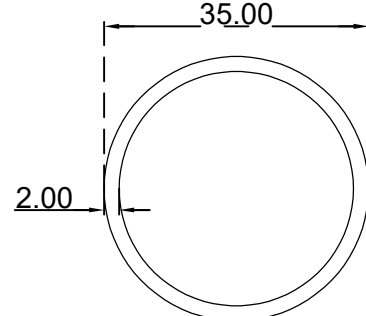
انبوب دائري مجوف (2*35) ملم الرقم التسلسلي للصنف: Y35X2 الوزن (Kg/m): 0.564
