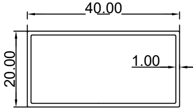
مستطيل (1*20*40) ملم الرقم التسلسلي للصنف: FG40X20X1 الوزن: 0.316:(Kg/m)
