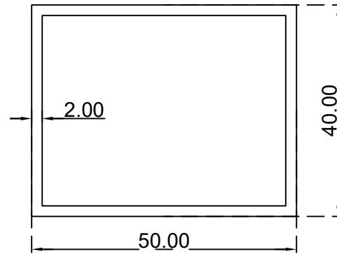
مستطيل (2*40*50) ملم الرقم التسلسلي للصنف: CAN022 الوزن: 0.946: (Kg/m)
