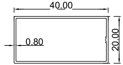
مستطيل (0.8*20*40) ملم الرقم التسلسلي للصنف: BLT3581 الوزن: 0.256:(Kg/m)
