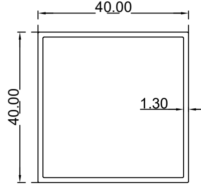
مربع (1.3*40*40) ملم الرقم التسلسلي للصنف: FG40X40X1.3A الوزن: 0.547: (Kg/m)
