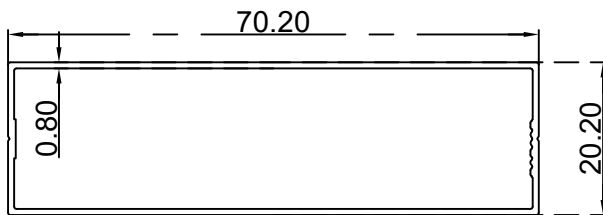
مستطيل (0.8*20.2*70.2) ملم الرقم التسلسلي للصنف: BLT3283 الوزن: 0.393: (Kg/m)
