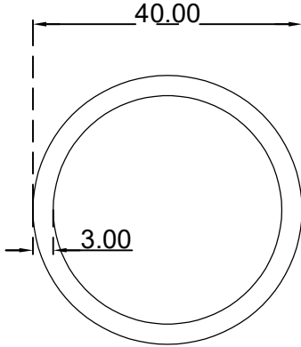
انبوب دائري مجوف (3*40) ملم الرقم التسلسلي للصنف: Y40X3B الوزن 0.952:(Kg/m)
