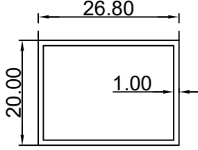
مستطيل (1*20*26.8) ملم الرقم التسلسلي للصنف: FG26.8X20X1 الوزن: 0.244:(Kg/m)
