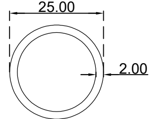
انبوب دائري مجوف (2*25) ملم الرقم التسلسلي للصنف: G25X2 الوزن (Kg/m): 0.393
