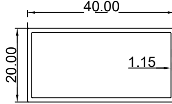
مستطيل (1*20*40) ملم الرقم التسلسلي للصنف: FG40X20X1.15 الوزن: 0.360:(Kg/m)
