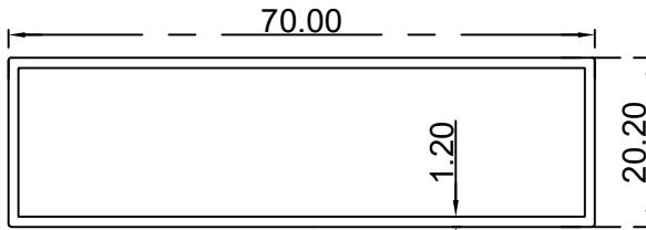
مستطيل (1.2*20.2*70) ملم الرقم التسلسلي للصنف: FG70X20.2X1.2 الوزن (Kg/m): 0.573
