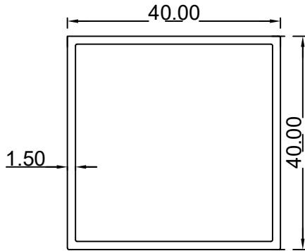
مربع 1.5*40*40 ملم الرقم التسلسلي للصنف: FG40X40X1.5 الوزن: 0.629: (Kg/m)
