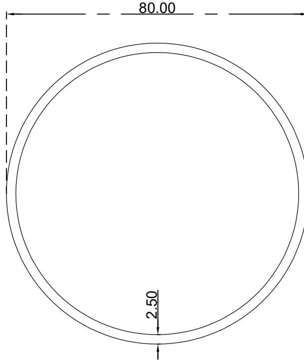
انبوب دائري مجوف (2.5*80) ملم الرقم التسلسلي للصنف: Y80X2.5A الوزن (Kg/m): 1.656
