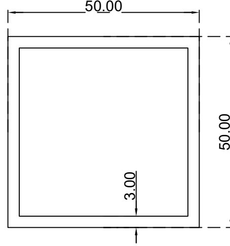
مربع (3*50*50) ملم الرقم التسلسلي للصنف: FG50X50X3 الوزن (Kg/m): 1.534
