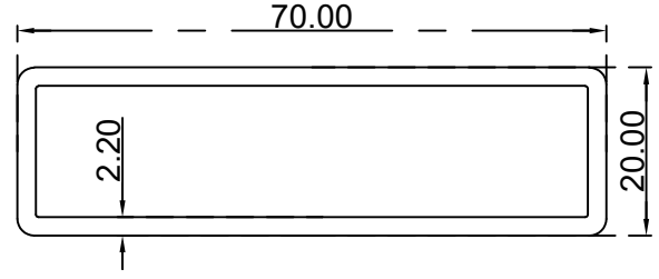
مستطيل (2.2*20*70) ملم الرقم التسلسلي للصنف: FG70X20X2.2C الوزن (Kg/m): 1.015
