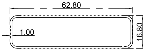
مستطيل (1*16.8*62.8) ملم الرقم التسلسلي للصنف: BLT3408 الوزن (Kg/m): 0.366
