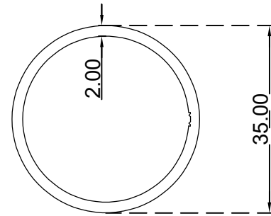
انبوب دائري مجوف (2*35) ملم الرقم التسلسلي للصنف: BLT3578 الوزن (Kg/m): 0.562
