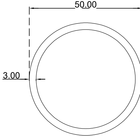
انبوب دائري مجوف (3*50) ملم الرقم التسلسلي للصنف: Y50X3 الوزن 1.205:(Kg/m)
