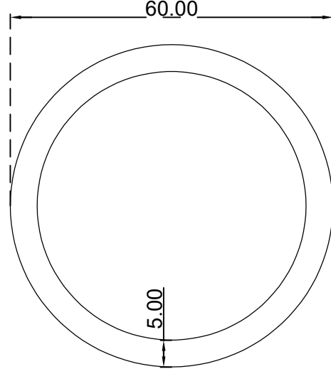
انبوب دائري مجوف (5*60) ملم الرقم التسلسلي للصنف: Y60X5 الوزن 2.350:(Kg/m)
