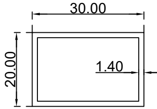
مستطيل (1.4*20*30) ملم الرقم التسلسلي للصنف: XSQ2030 الوزن: 0.353:(Kg/m)
