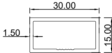
مستطيل (1.5*15*30) ملم الرقم التسلسلي للصنف: FG30X15X1.5 الوزن: 0.339:(Kg/m)
