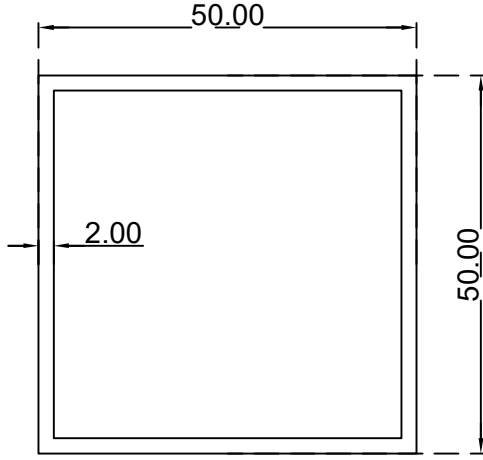
مربع (2*50*50) ملم الرقم التسلسلي للصنف: SA5001 الوزن (Kg/m): 1.041
