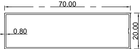
مستطيل (0.8*20*70) ملم الرقم التسلسلي للصنف: BLT3580 الوزن (Kg/m): 0.386
