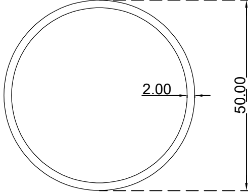
انبوب دائري مجوف (2*50) ملم الرقم التسلسلي للصنف: Y50X2 الوزن 0.820:(Kg/m)
