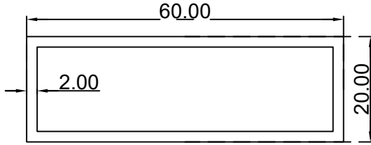
مستطيل (2*20*60) ملم الرقم التسلسلي للصنف: FG60X20X2 الوزن (Kg/m): 0.827
