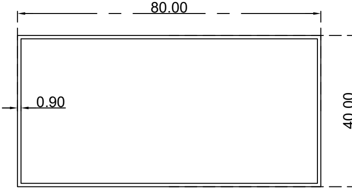
مستطيل (0.9*40*80) ملم الرقم التسلسلي للصنف: YH-ME1042 الوزن (Kg/m): 0.578
