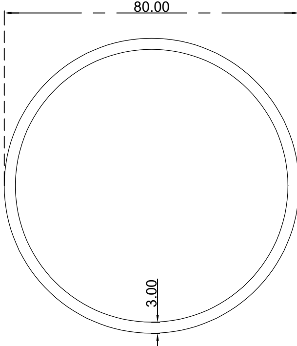
انبوب دائري مجوف (3*80) ملم الرقم التسلسلي للصنف: Y80X3A الوزن (Kg/m): 1.974
