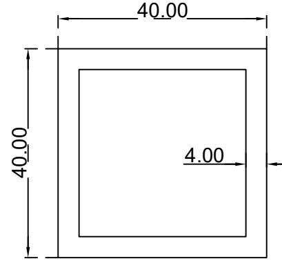
مربع (4*40*40) ملم الرقم التسلسلي للصنف: FG40X40X4.0 الوزن: 1.566: (Kg/m)
