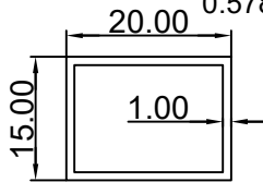
مستطيل (1*15*20) ملم الرقم التسلسلي للصنف: FG20X15X1 الوزن (Kg/m): 0.180
