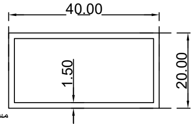
مستطيل (1.5*20*40) ملم الرقم التسلسلي للصنف: FG40X20X1.5 الوزن: 0.465:(Kg/m)
