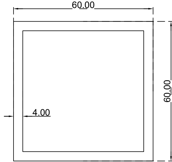
مربع (4*60*60) ملم الرقم التسلسلي للصنف: FG60X60X4 الوزن (Kg/m): 2.440
