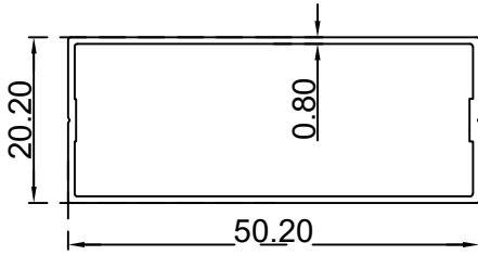
مستطيل (0.8*20.2*50.2) ملم الرقم التسلسلي للصنف: BLT3284 الوزن: 0.306: (Kg/m)
