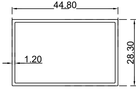
مستطيل (1.5*30*30) ملم الرقم التسلسلي للصنف: FG44.8X28.3X1.2 الوزن: 0.463: (Kg/m)
