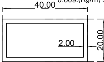
مستطيل (2*20*40) ملم الرقم التسلسلي للصنف: FG40X20X2D الوزن: 0.609:(Kg/m)
