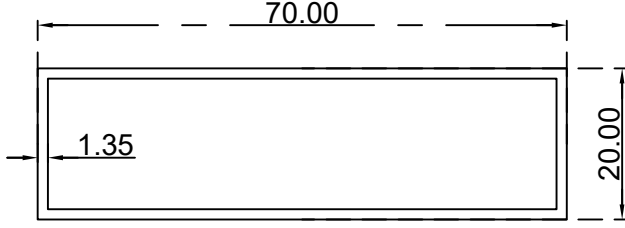
مستطيل (1.35*20*70) ملم الرقم التسلسلي للصنف: FG70X20X1.35 الوزن (Kg/m): 0.641
